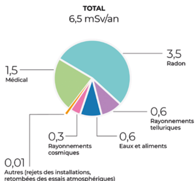
Figure 13. Exposition moyenne aux rayonnements ionisants de la population en France (mSv/an) (Source IRSN 2021)
