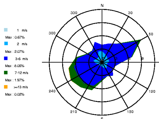
Figure 8 : rose des vents générale – Station Météo-France de Tours – 2018-2022 (5 ans)
