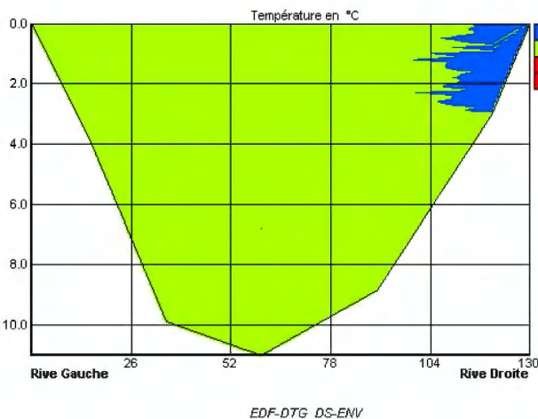
Figure 19 : Transects de température en aval du CNPE de Tricastin réalisés en 2006.
