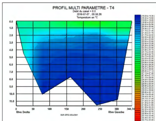
Profil de température à 0,5 km en aval des rejets
