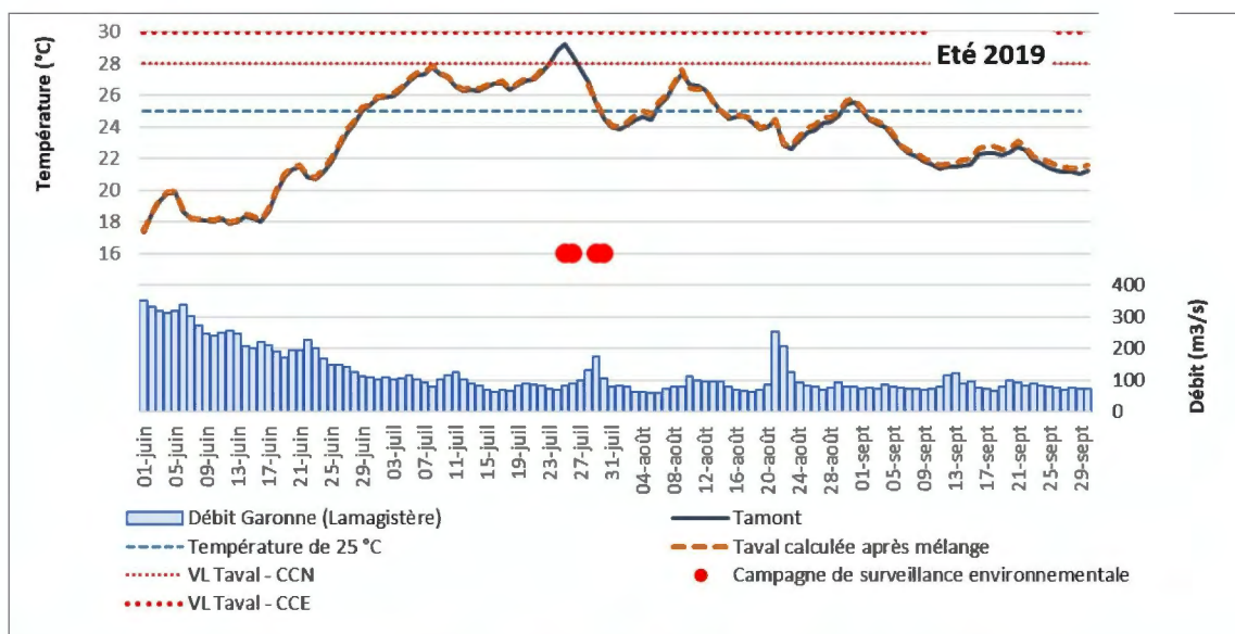
Figure 25 : Caractéristiques de l'été 2019 de la Garonne au CNPE de Golfech
