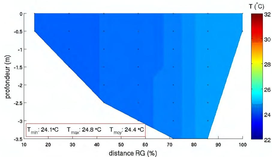
Figure 8 : Profils thermiques en aval du CNPE de Bugey le 22 août 2009 (débit moyen du Rhône de 364 m 3 /s, échauffement moyen de 1,1 °C après mélange).
