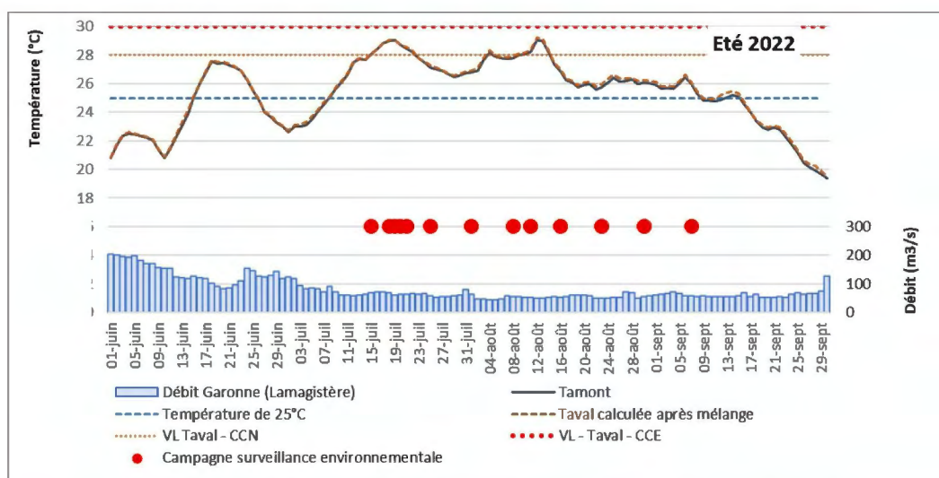
Figure 26 : Caractéristiques de l'été 2022 de la Garonne au CNPE de Golfech
