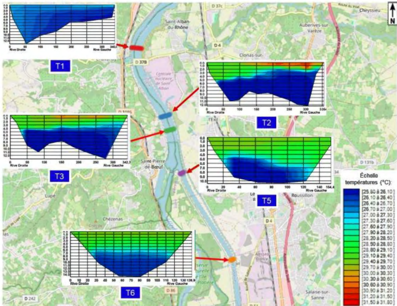
Figure 18 : Profils de température (°C) mesurés lors de la campagne du 18/08/2025
