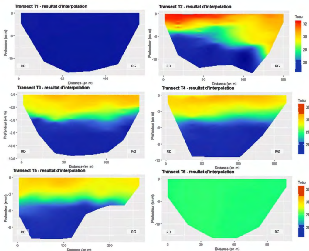
Figure 22 : Profils de température (°C) mesurés lors de la campagne du 10/08/2022
