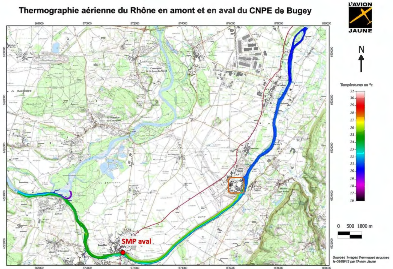
Figure 9 : Thermographie aérienne du panache thermique du CNPE de Bugey le 8 septembre 2012
