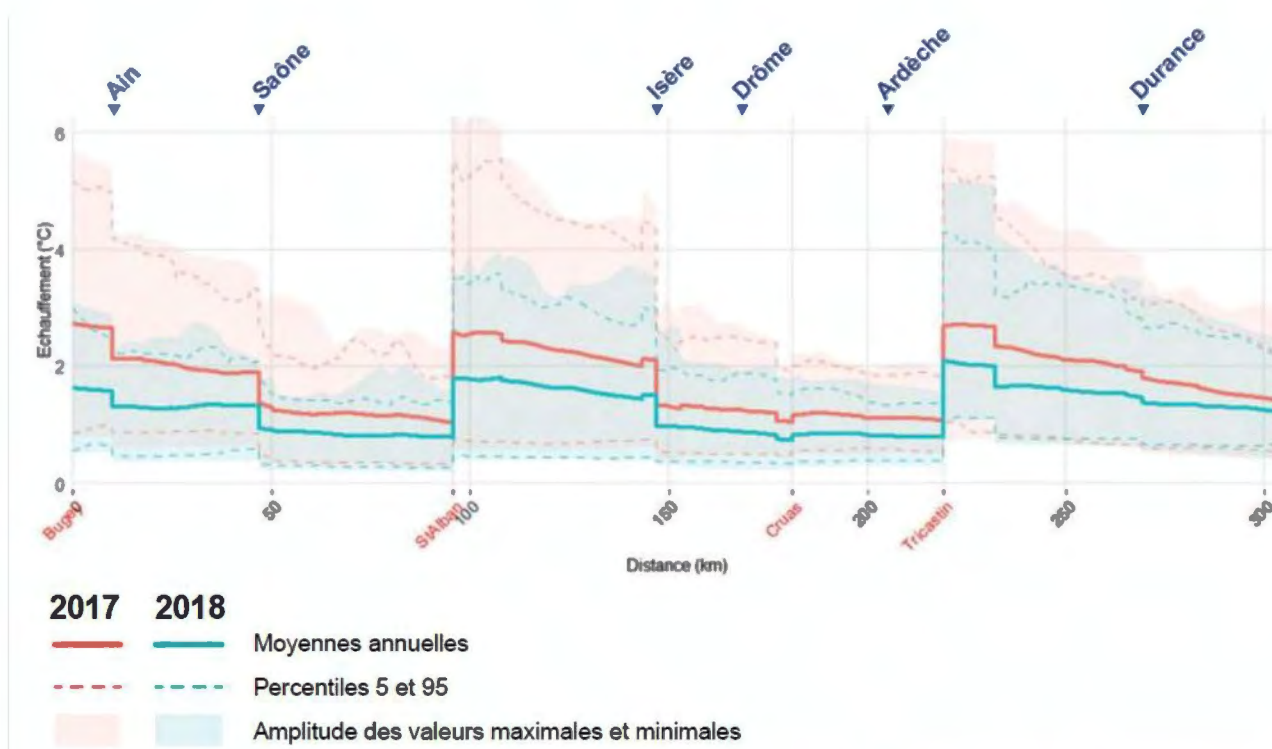
Figure 24 : Valeurs moyennes annuelles des échauffements résiduels calculés le long du linéaire du Rhône pour les années 2017 et 2018
