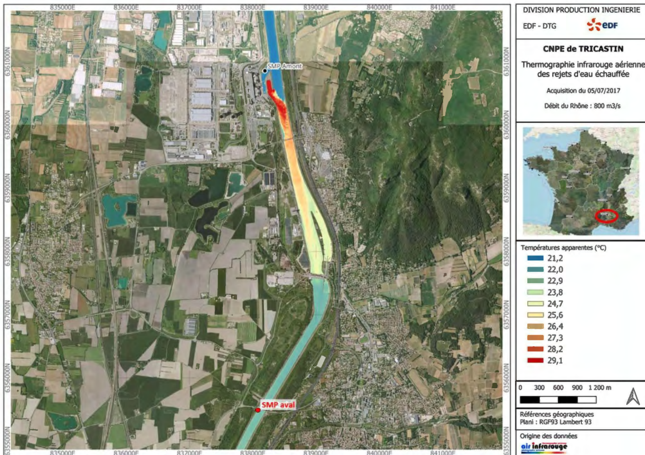
Figure 20 : Thermographie réalisée le 5 juillet 2017 en aval du CNPE du Tricastin. Le débit du Rhône est d'environ 790 m 3 /s, le CNPE fonctionne à 75% de sa puissance nominale.
