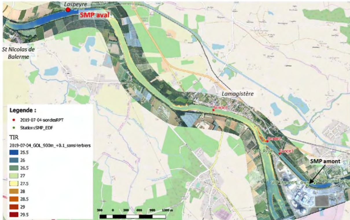
Figure 5 : Thermographie aérienne du panache thermique du CNPE de Golfech durant l'été 2019.
