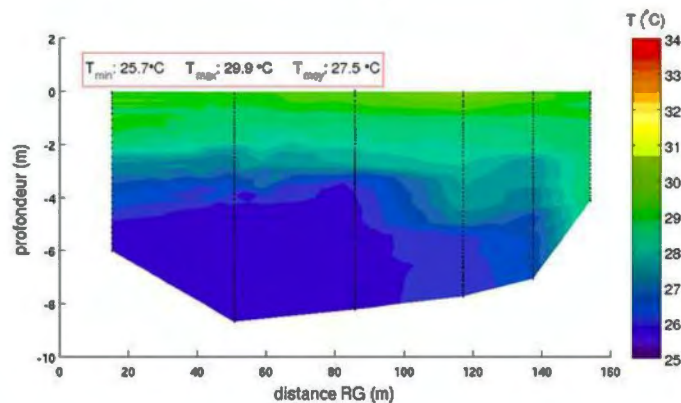
Figure 13 : Transects de température en aval du CNPE de Saint-Alban le 7 juillet 2015 (débit du Rhône de 600 m 3 /s et température du Rhône de 25,5 °C en amont). Le CNPE fonctionne à pleine puissance et l'échauffement calculé après mélange est de 1,9 °C.
