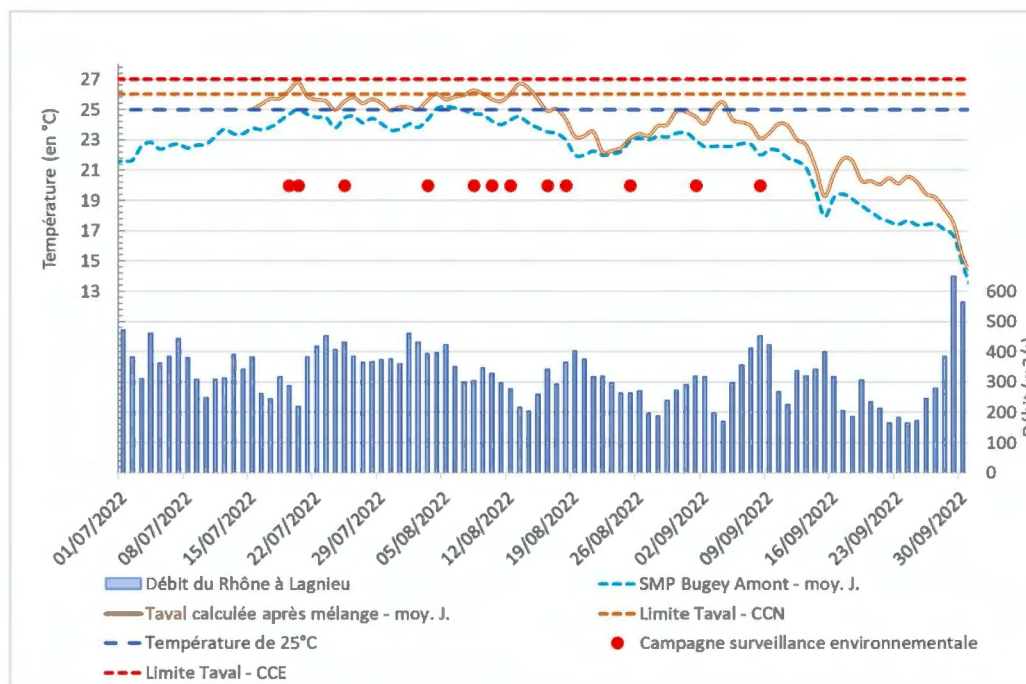
Figure 27 : Caractéristiques de l'été 2022 du Rhône au CNPE de Bugey
