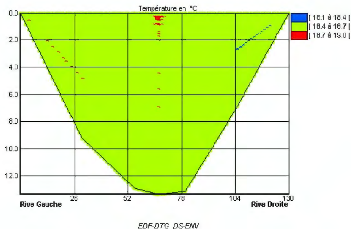
Figure 19 : Transects de température en aval du CNPE de Tricastin réalisés en 2006.
