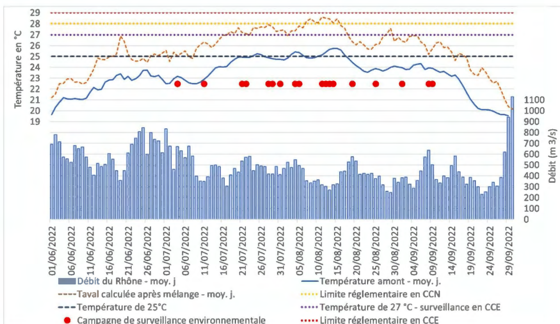
Figure 28 : Caractéristiques de l'été 2022 du Rhône au CNPE de Tricastin
