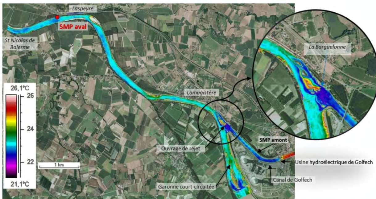
Figure 1 : Thermographie aérienne du panache thermique du CNPE de Golfech durant l'été 2006. À gauche : vue globale ; à droite : zoom sur la zone de rejet (conduite multipores).
