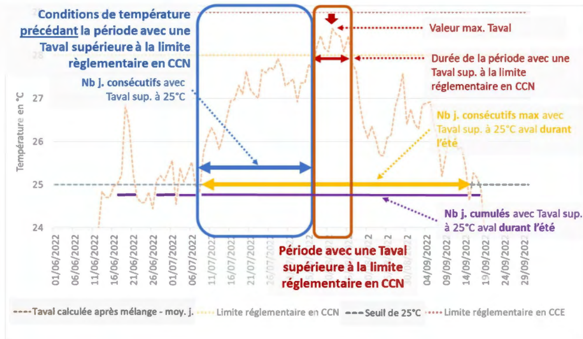
Figure 29 : Conditions de température avant et pendant le passage en SE – clef de lecture
